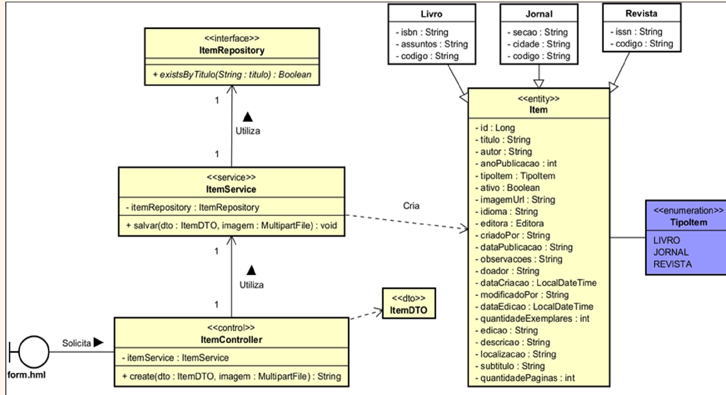
Figura 2 - Diagrama de Classe - Criação do item
