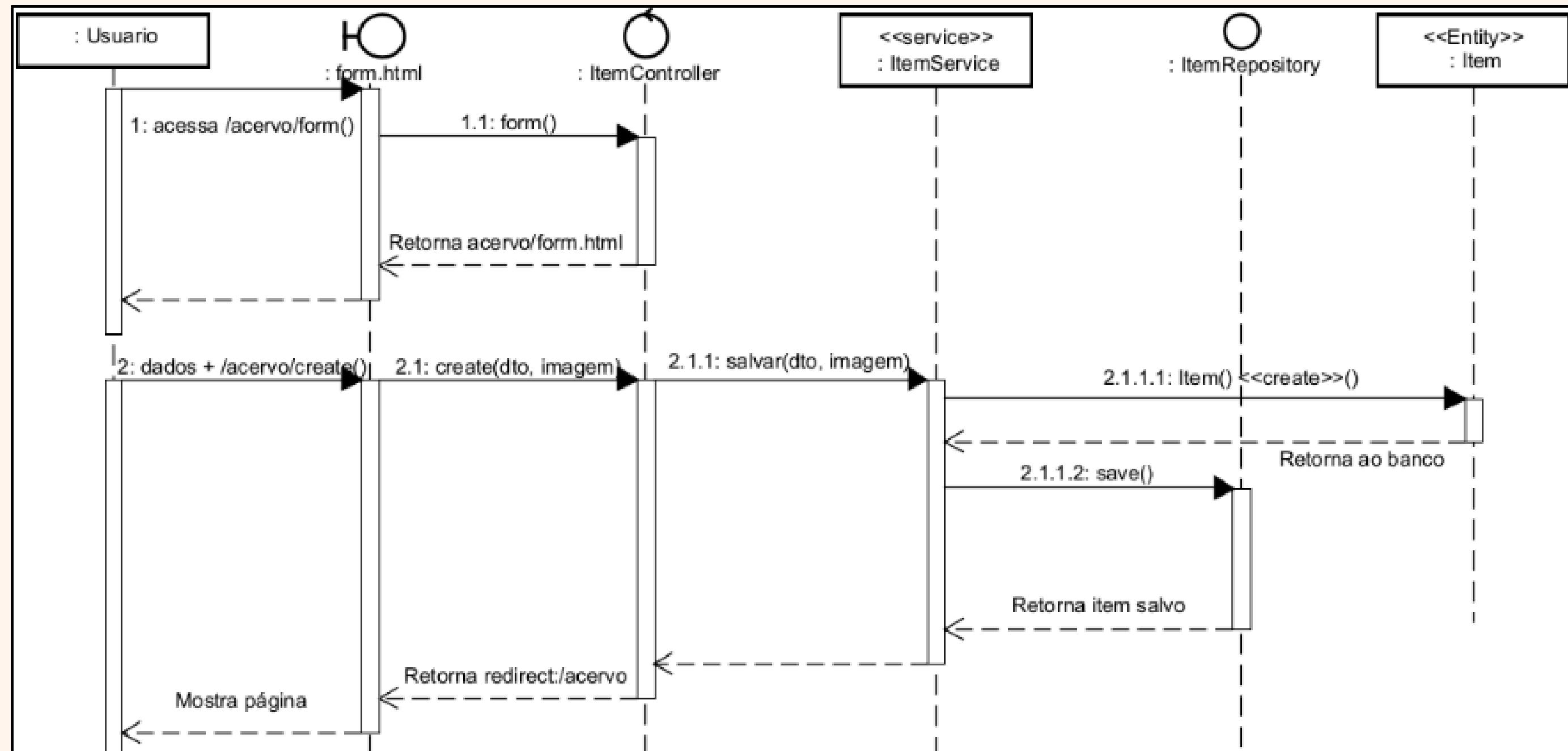
Figura 3 - Diagrama de Sequência - Criando um Item
